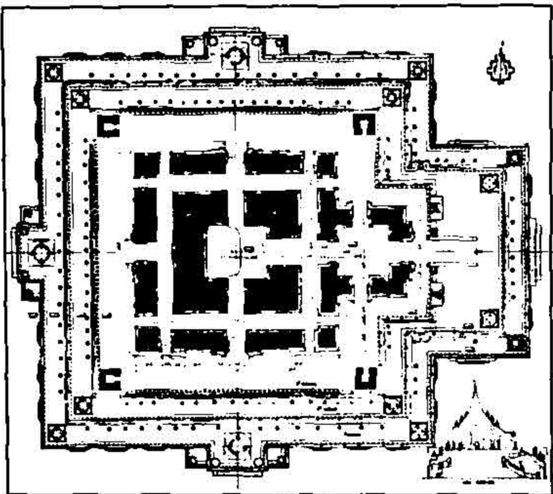
သမ္ဗညဘုရား ဒုတိယထပ် ပန္နက်ပုံ
