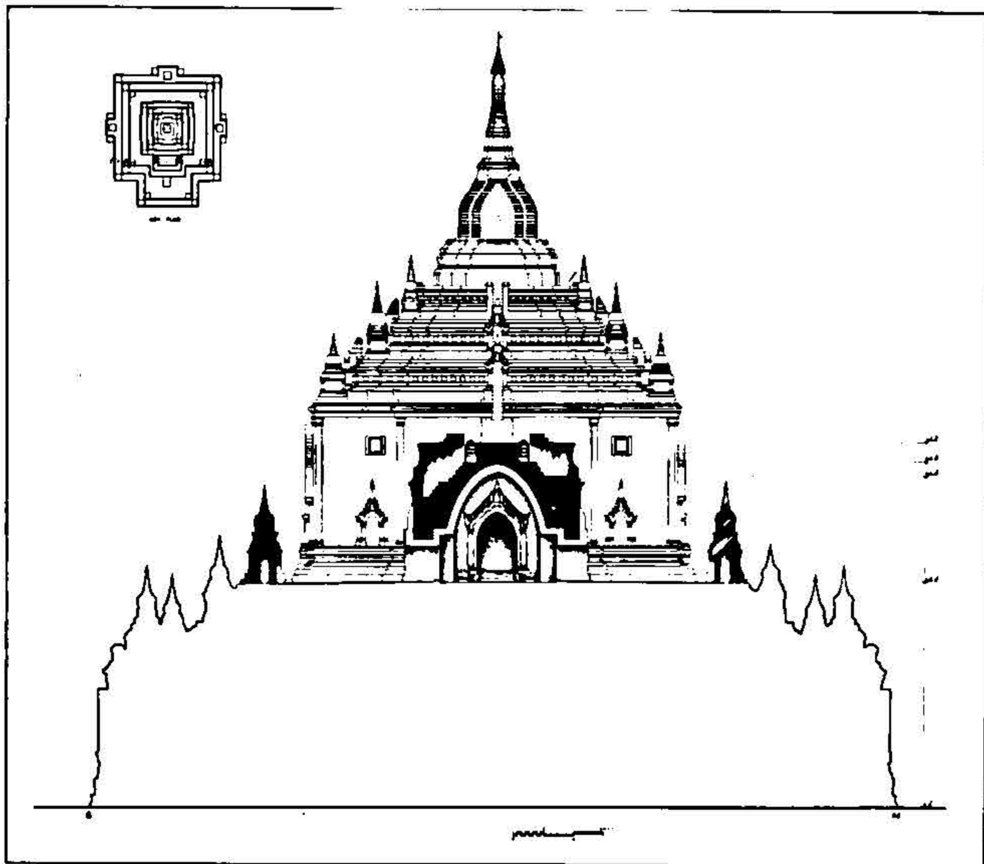
သဗ္ဗညုဘုရား တတိယထပ်ပစ္စယံ ဖြတ်ပိုင်းပုံ
