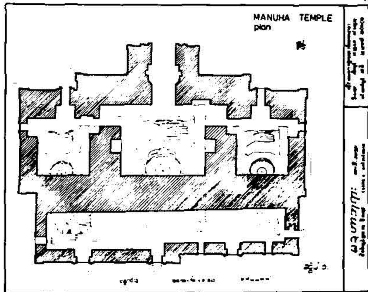
မနုဟာဘုရားပန္နက်ပုံ
