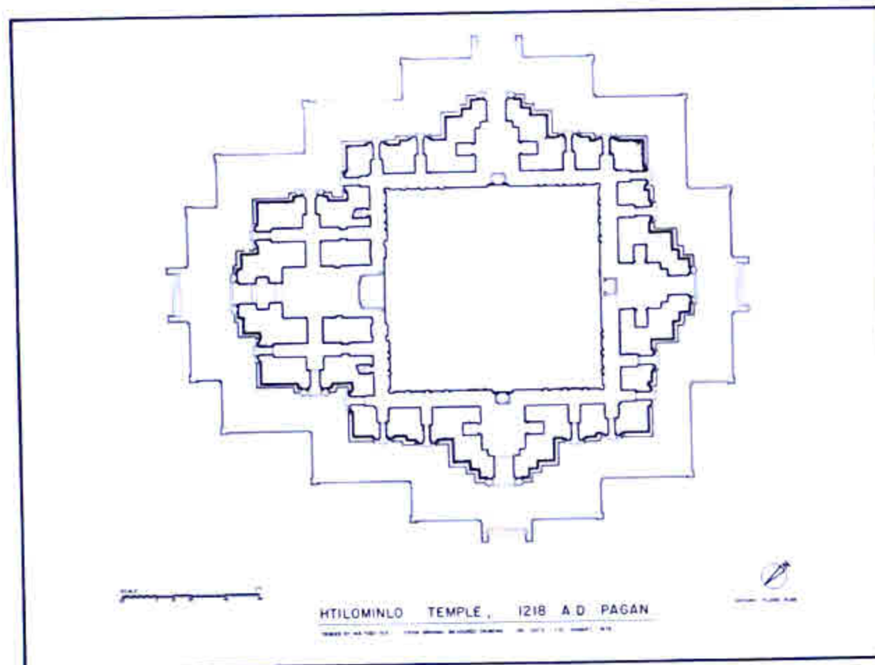
ထီးလိုမင်းလိုဘုရား မြေညီထပ် ပန္နက်ပုံ
