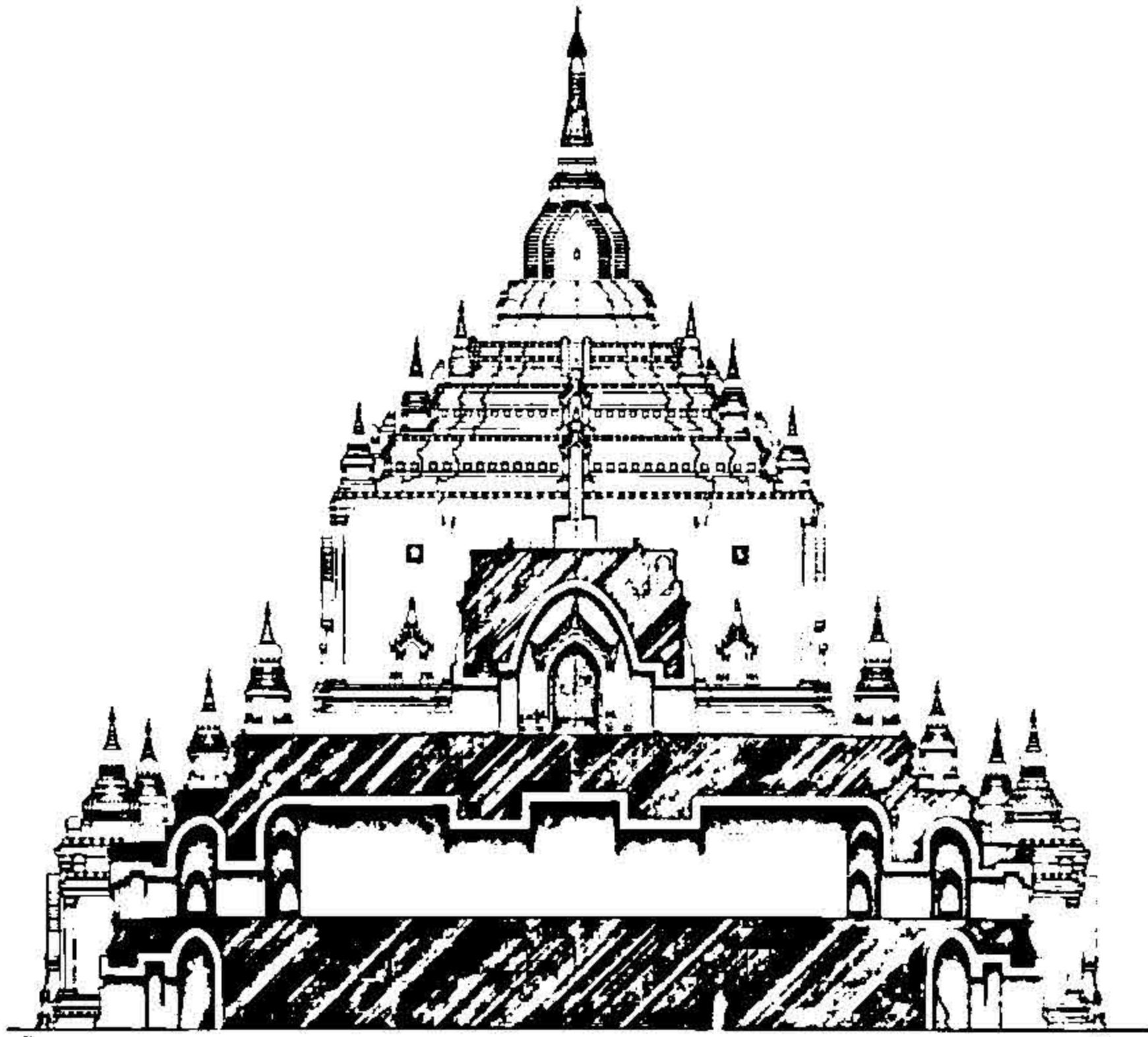
သဗ္ဗညုဘုရား တောင်-မြောက် ဖြတ်ပိုင်းပုံ
