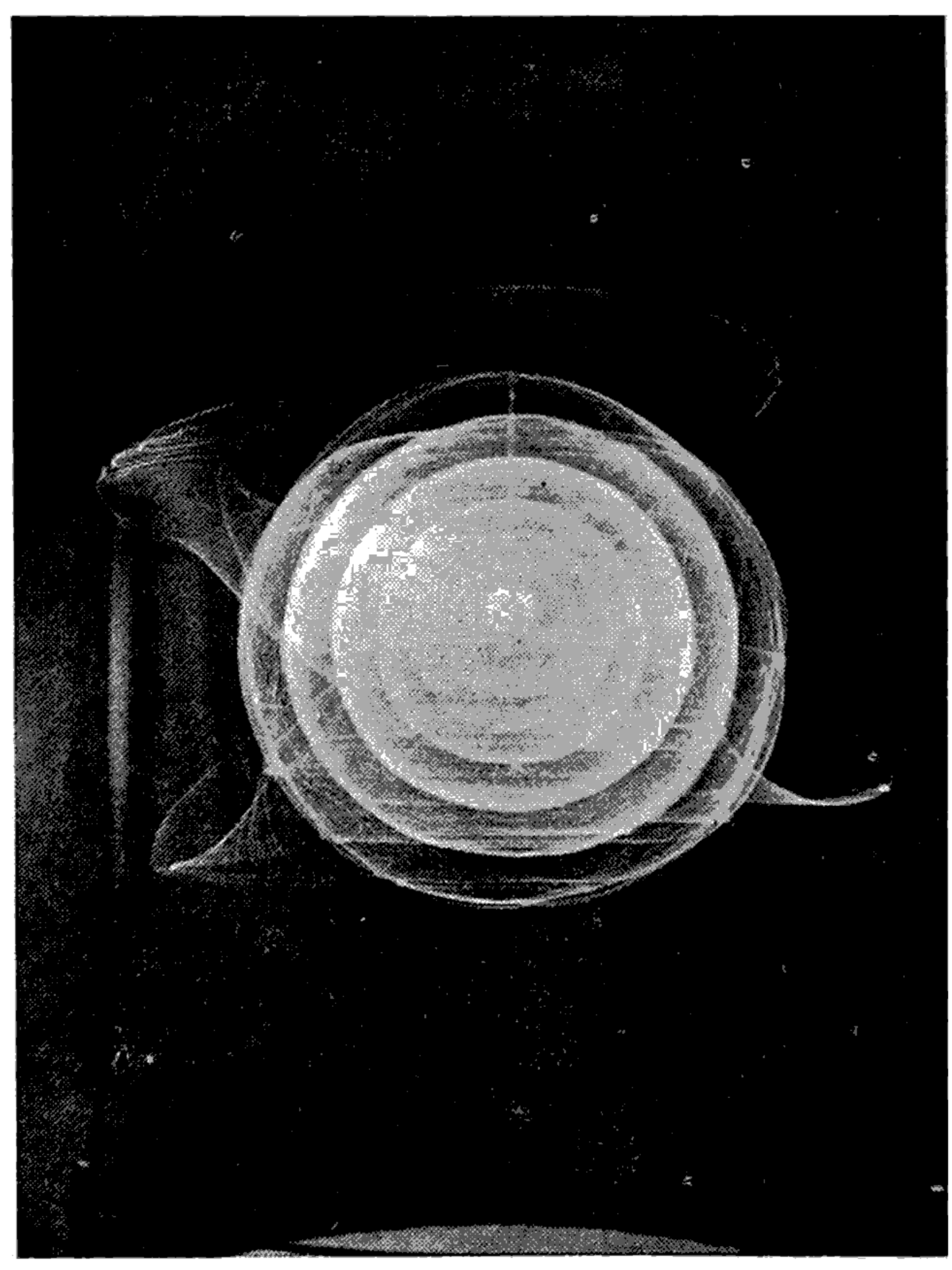
ယူရေးနီးယမ်း အနုမြူ လှုပ်ရှား လှည့်ပတ်နေပုံ ဖြစ်သည်။ အနုမြူ စွမ်းအင် ထုတ်လုပ် အသုံးချရေးတွင် ယူရေးနီးယမ်းသည် အထူး အသုံးဝင် အရေးကြီးသည်။
