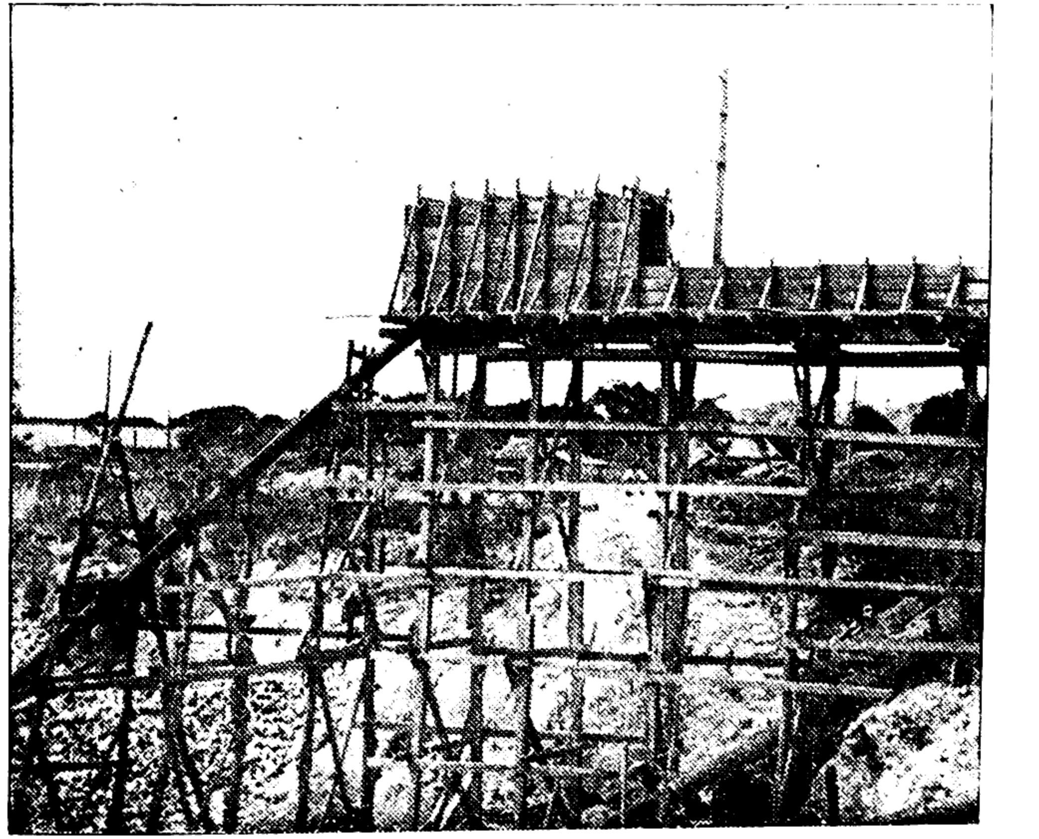
ထားဝယ်ခရိုင် ကံပေါက် သတ္တုတူးလုပ်ငန်းတွင် သတ္တုများ စုပ်နေစဉ်
