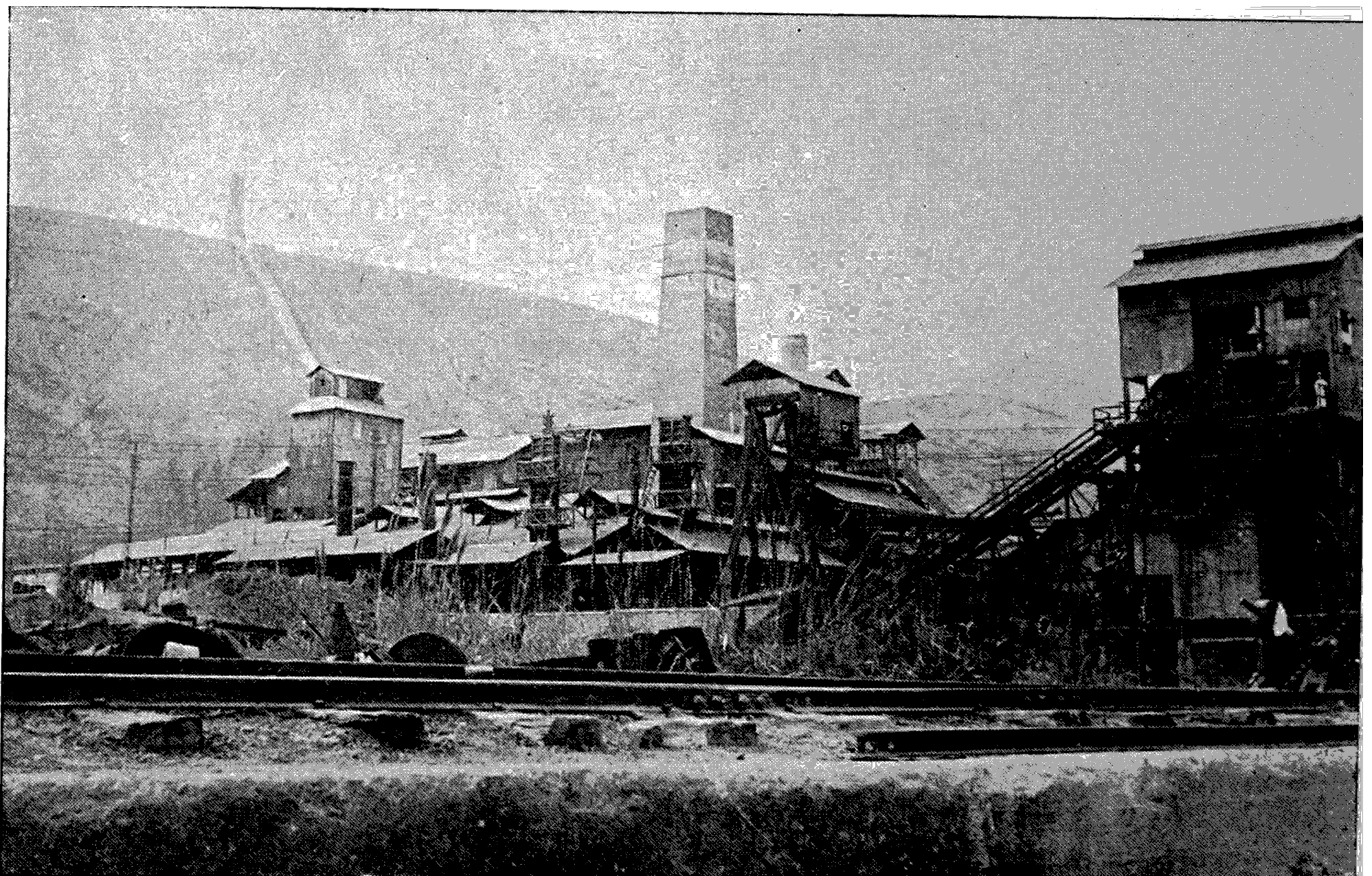
နမူတူ ဘော်ချက်စက်ရုံ၏ ရှုခင်းပုံဖြစ်သည်။ စက်ရုံမှ ထုတ်သော ခဲအဆိပ်ငွေ့များကို မရွှေ့မိကြစေရန် ခဲအငွေ့ထုတ်ခေါင်းတိုင်ကို တောင်ပေါ်၌ သီးခြား တည်ဆောက်ထားရသည်။
