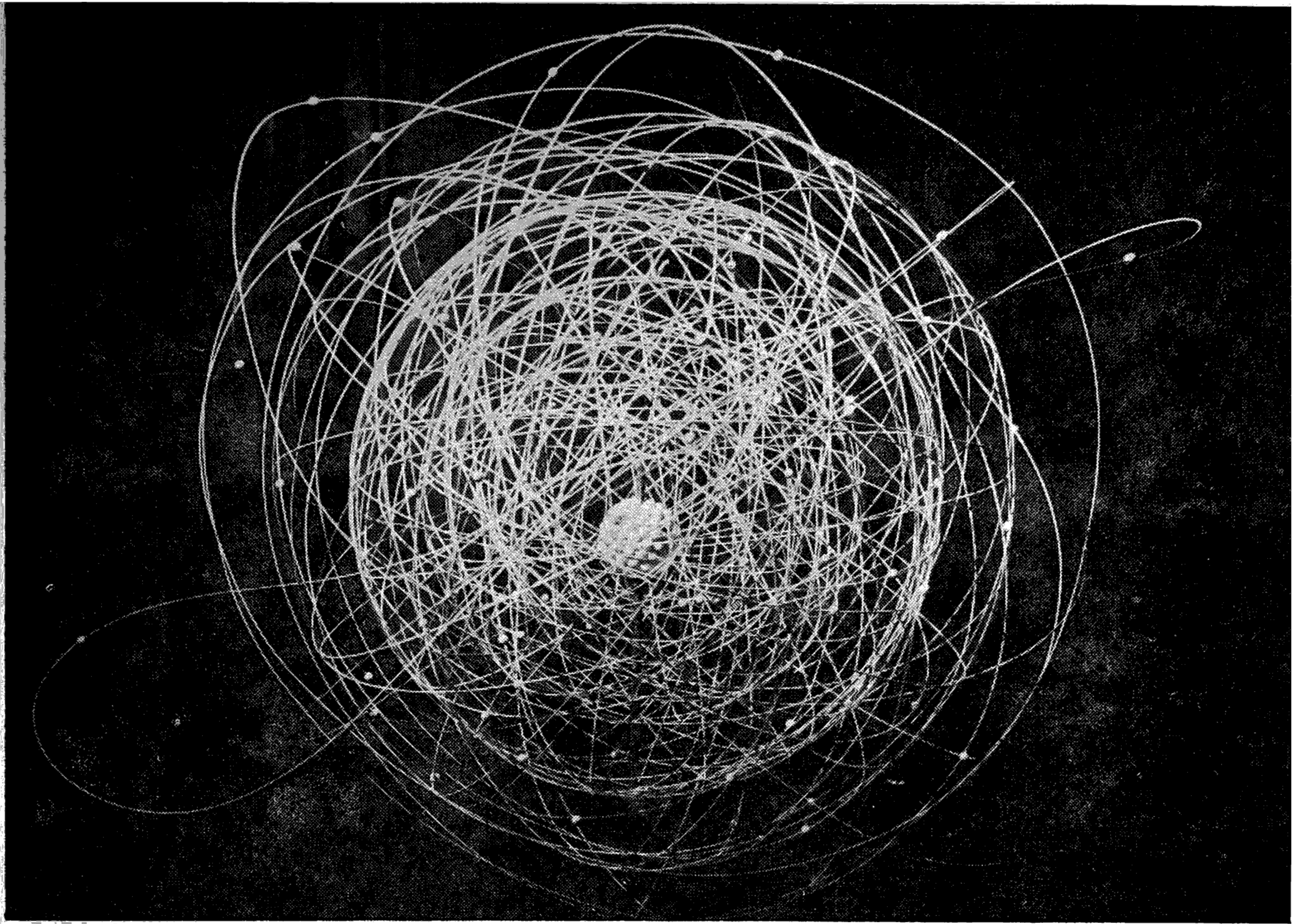
ယူရေးနီးယမ်း အနုမြူတခု၏ ဖွဲ့စည်းနေဟန်
